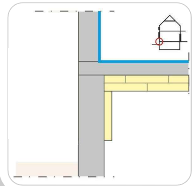
- Dämmung in zwei Schichten versetzt
